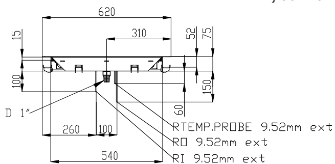
Zij aanzicht
